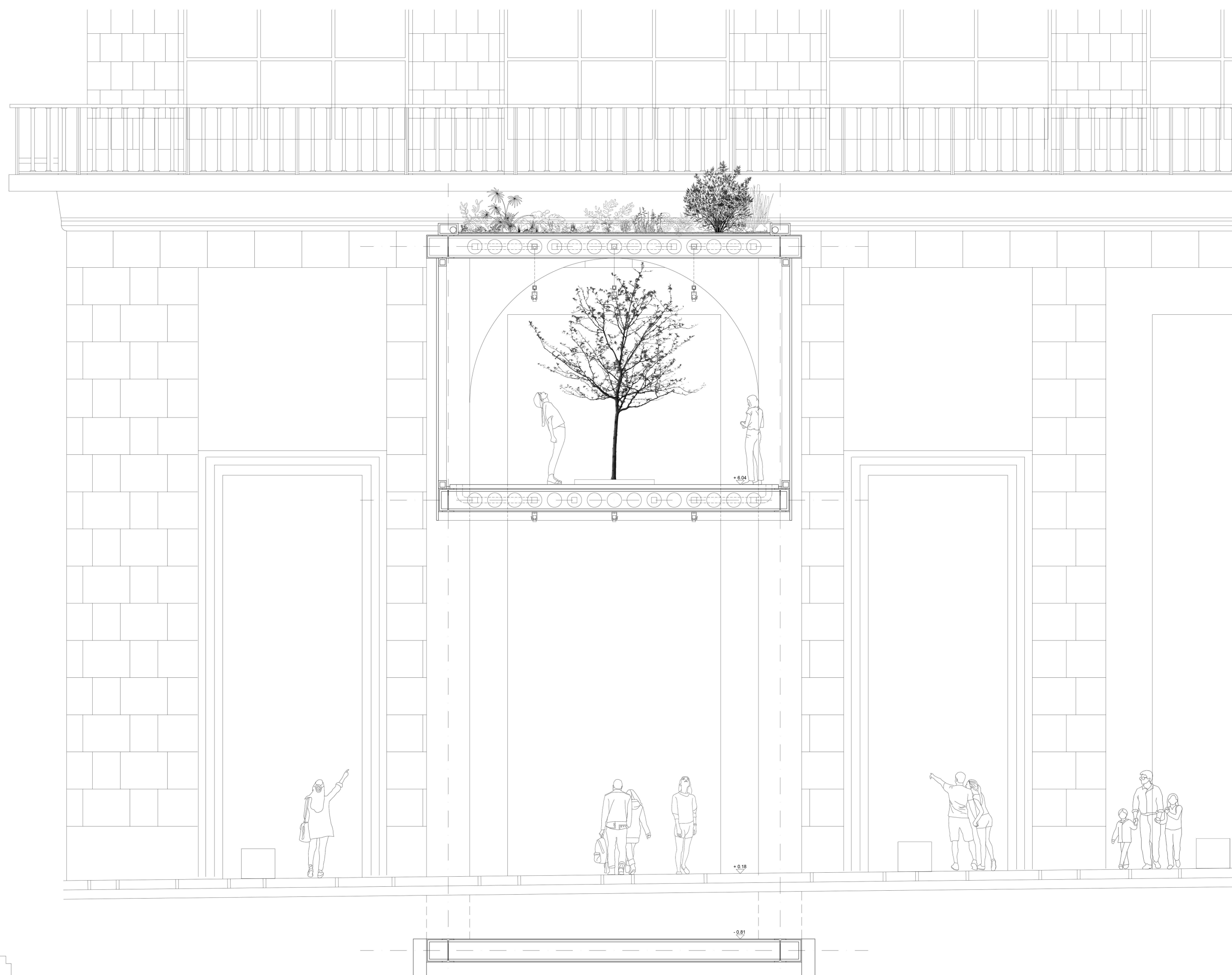
SEZIONE E - DETTAGLIO COSTRUTTIVO 1:50
